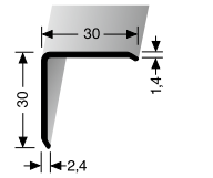
273 U ECKSCHUTZWINKEL CORNER GUARD
