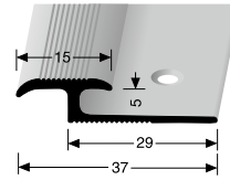
292 EINFASSPROFILE EDGE TRIM
