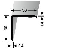
273 SK* ECKSCHUTZWINKEL CORNER GUARD
